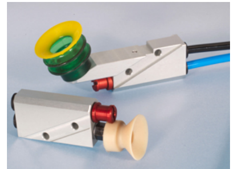
SPM-Modul mit pneumatischer Vakuumpumpe
