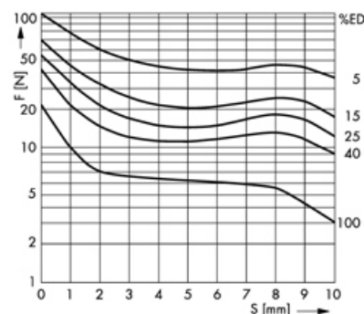
Angepasste Kraft-Weg-Kennlinie
